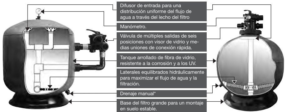
Filtros de fibra de vidrio de montaje lateral Waterco.
